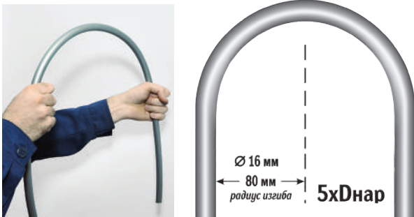
Минимальный радиус изгиба труб КОНТУР G-RAY
